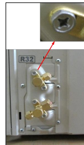
※アプセットボルトの使用例
