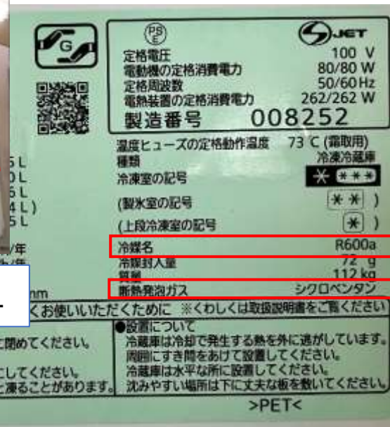
銘板シールの一例 (冷媒・断熱発泡ガスの種類の表示例)
